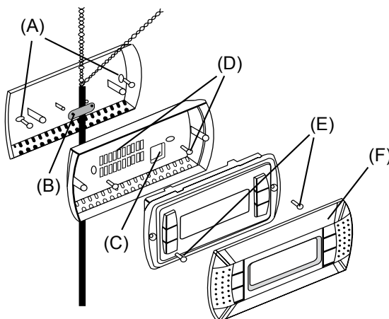
Obr. 3.1 montáž ovládacího modulu na stěnu
