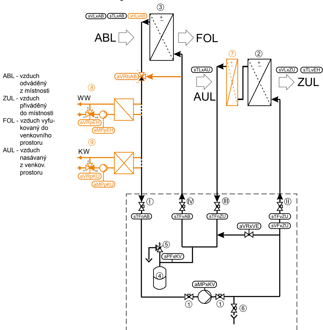
funkční schéma hydraulické jednotky s dodáváním energie
