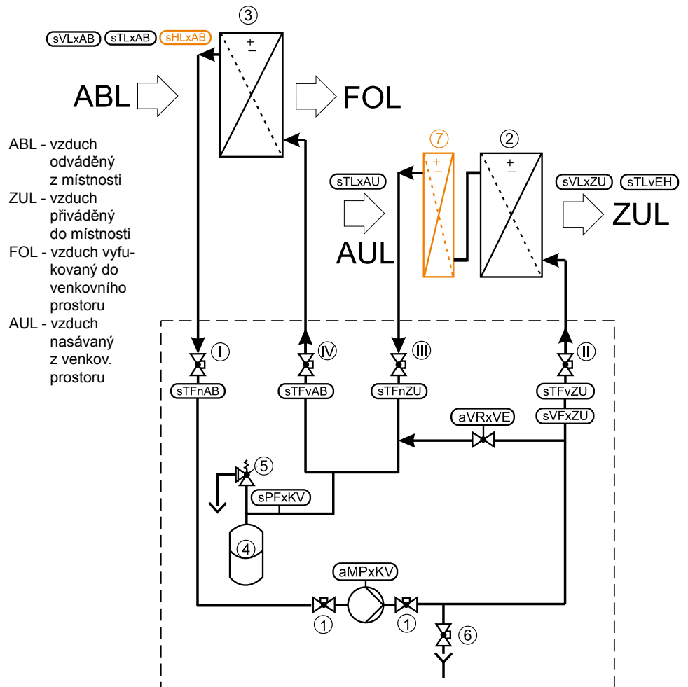
funkční schéma hydraulické jednotky
